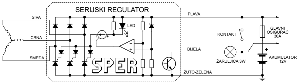
Slika 2 - Spoj regulatora (6/8 žica):
